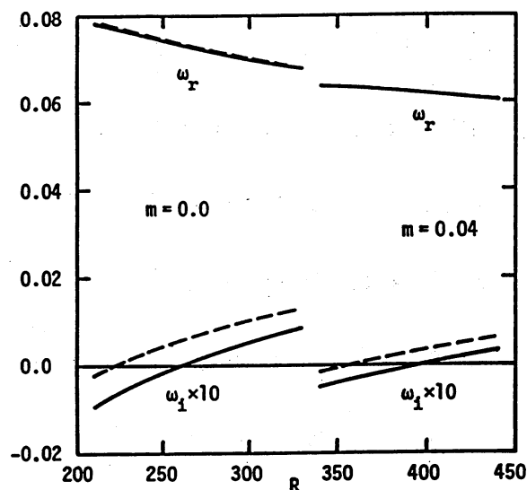
図1. T-S不安定の最大増幅率と補正解 ( \gamma = 1.0 )
