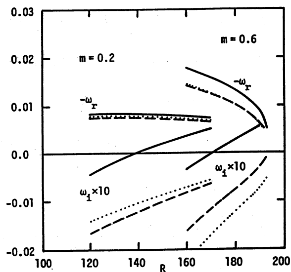
図3. S-C不安定の最大増幅率と補正解 ( \gamma = 1.0 )
