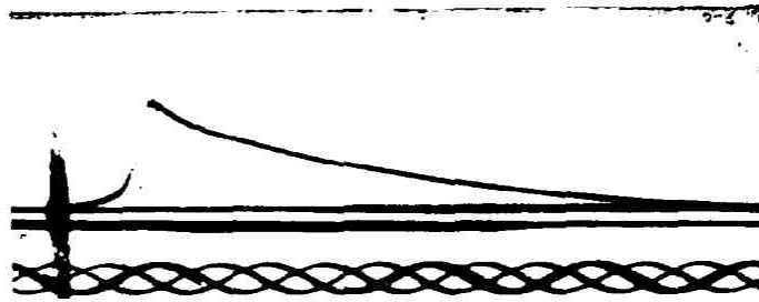
Fig. 5. No. 55. H_2:O_2=8:1 , P=8 cmHg (容器 No. 1, 薄膜 I.)
