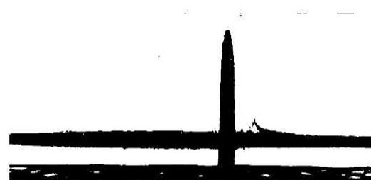
Fig. 13. No. 151. \text{H}_2:\text{O}_2=2:1 , P=7\text{ cmHg}
