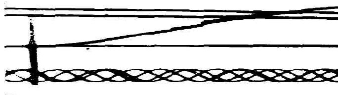
Fig. 9. No. 75. H_2:O_2=1:8 , P=7 cm (容器 No. 8, 薄膜)
