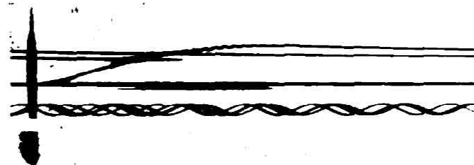
Fig. 8. No. 73. H_2:O_2=1:8 , P=8 cm (容器 No. 5, 薄膜 I.)
