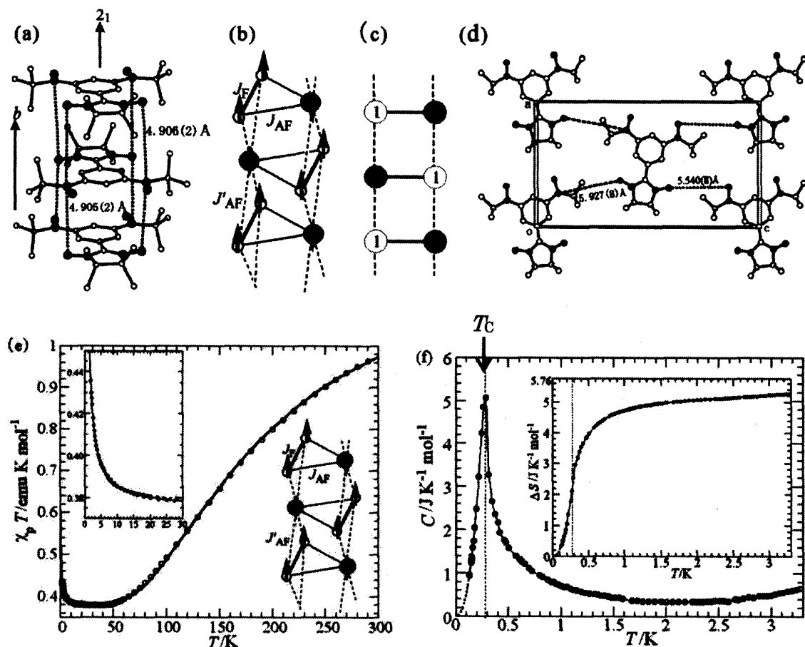
図9 (a) PNNBNO 結晶の b 軸方向に形成される鎖状構造。黒丸と灰色丸はそれぞれ t\text{BuNO} と \text{NN} の \text{NO} 部位を表している。点線は分子間接近を表す。(b) (a)の磁性モデル。白丸および灰色の丸はそれぞれ t\text{BuNO} と \text{NN} に対応し、いずれも S = 1/2 を表す。 J_F , J_{AF} はそれぞれ分子内の強磁性および反強磁性相互作用を、 J'_{AF} は分子間反強磁性相互作用を表す。(c) J_F \rightarrow \infty の極限では、(b)はフェリ磁性梯子となる。(d) PNNBNO の結晶構造の ac 面投影図。破線は鎖間分子接近を表す。(e) PNNBNO の \chi_p T の温度依存性。挿入図：低温部の拡大。(f) PNNBNO の磁気比熱の温度依存性。挿入図：エントロピー変化量。
