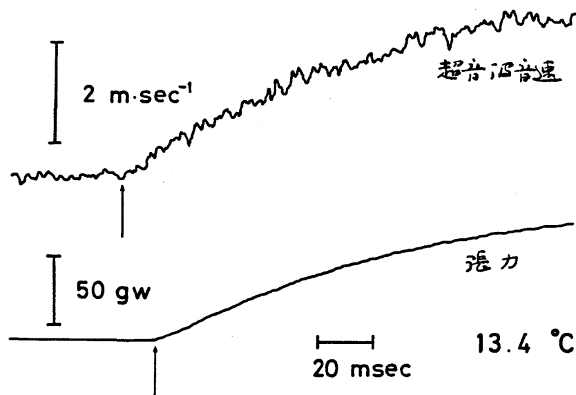
Fig. 1. 弛緩状態から弾性状態への遷移過程における音速および張力の時間変化の立ち上がり
