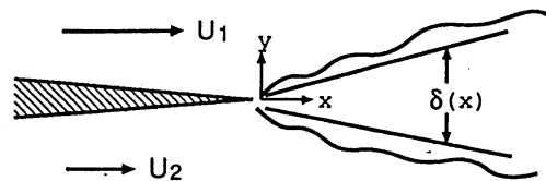
図 14. 超音速混合層
