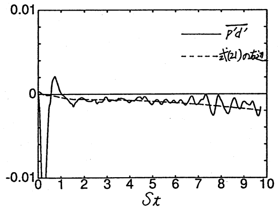
図 10. \overline{p'd'} と式 (21) の右辺の比較 (SH1)
