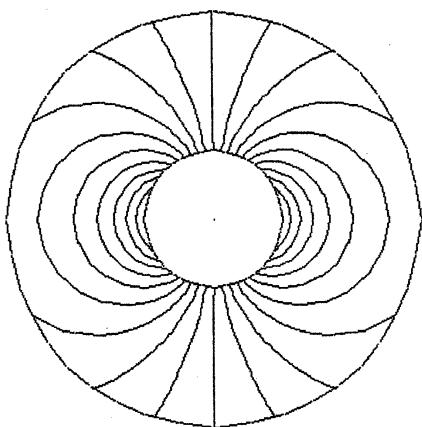
図 7: 数値解 u_0^{(3)}
