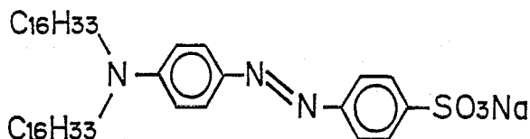
Azo form
