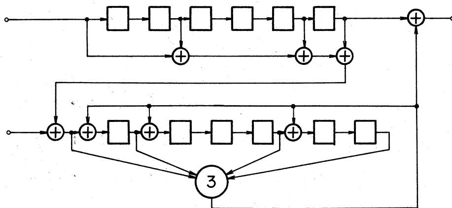
第3図 復号器
