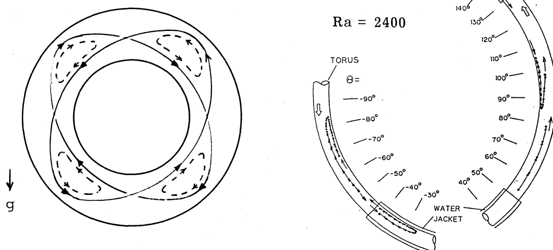
図 2. (a) 3 次元流の発生 (b) 流れの可視化の例
