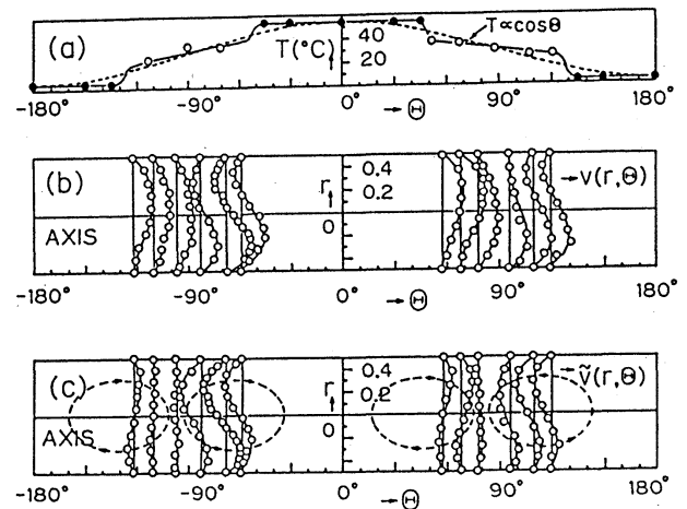
図 3. 速度の L D V 測定
