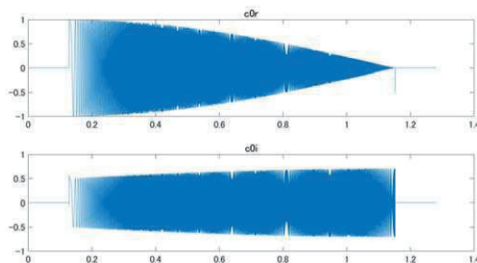
図 13 Interpolation
