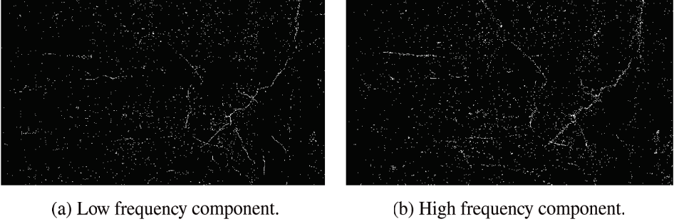
図 16 Binary image
