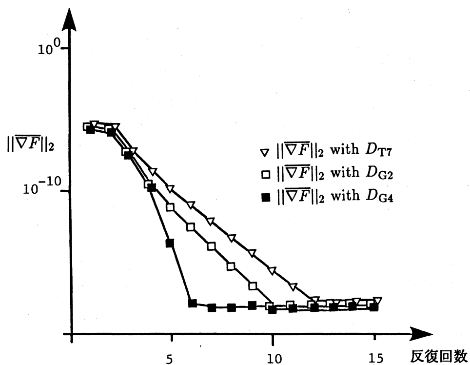
図 3.(b) 勾配 \nabla \bar{F} の 2 ノルム.
