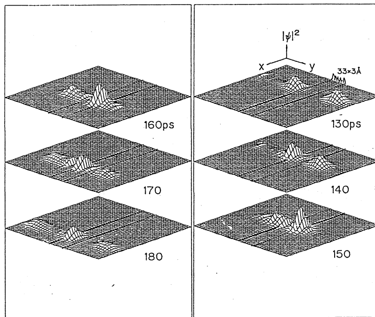
Figure 2: (a) 波束が干渉計で分割される様子、(b) 同じく重ね合わせが生じる様子を示すダイナミックスの解。ともに、ブラッグ条件が満たされる場合。
