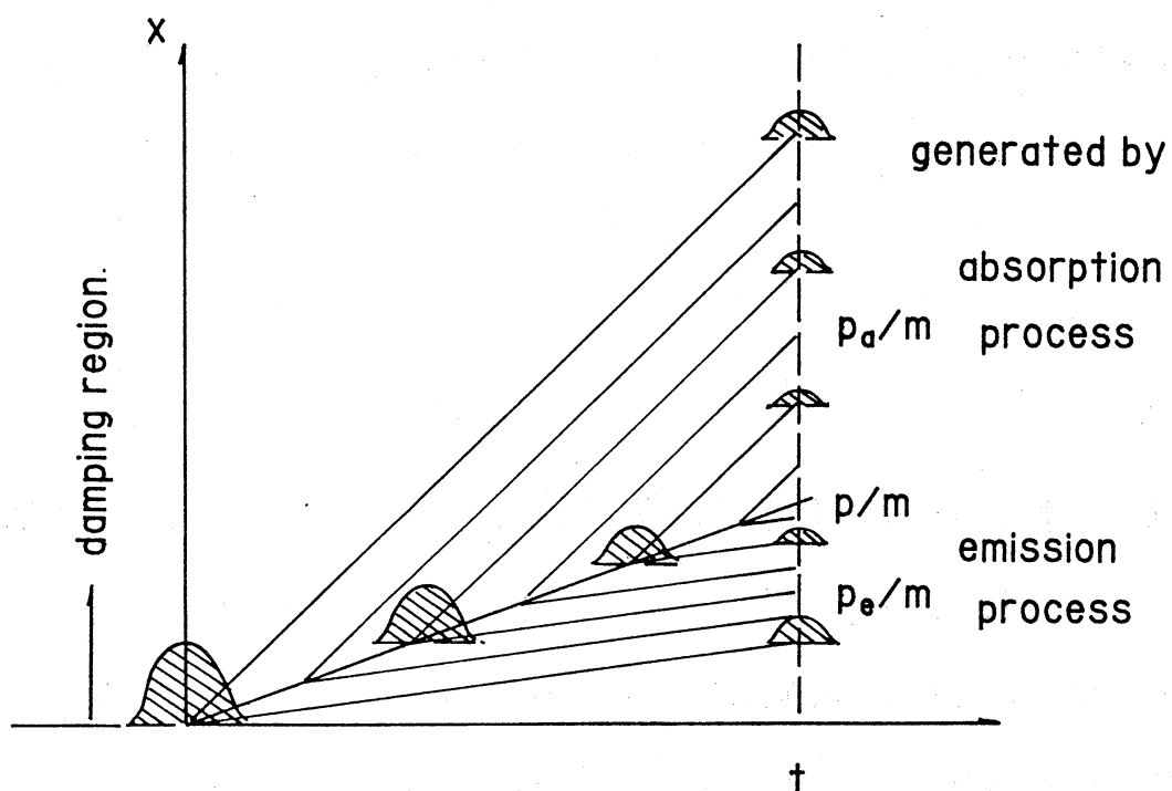
Figure 4: 初期波束が非弾性散乱によって小さな波束を連続して発生する様を概念的に示す図。
