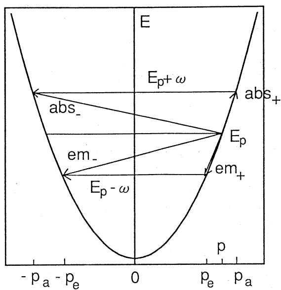
Figure 3: 光学フォノンによる非弾性散乱の素過程。
