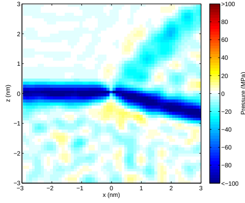
(c) p_{tt} .
