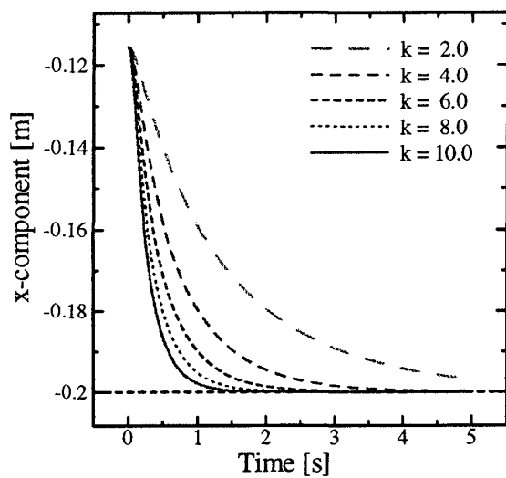
図 5: スチックネル k を変化したときの 手先位置 (x, y) の x の過渡応答.
