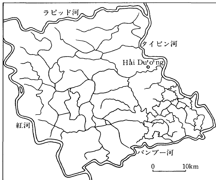
図4 中央デルタの水文環境。全ての川は紅河などの大河からの入水口をもたない
