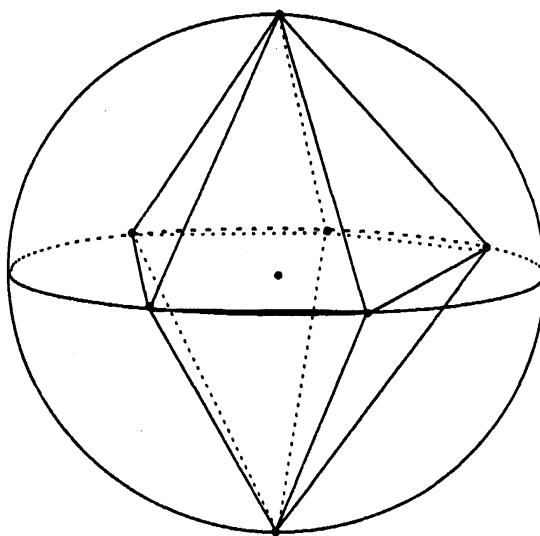
Fig. 3. \mathbb{R}^3 における唯1つの 8-point isosceles set
