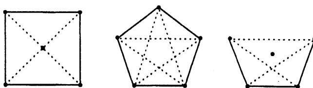
Fig. 3. \mathbb{R}^3 における唯1つの 8-point isosceles set
