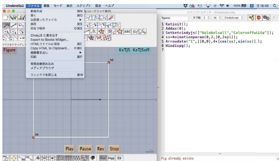
図 2. K E TCindyJS の画面と Script エディタ
