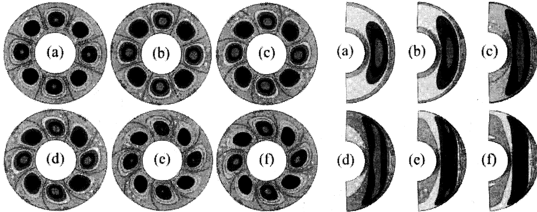
図 3: 臨界モード ( R = R_c ) の, 赤道面 ( \theta = 90^\circ ) における速度場の動径成分 u_r と子午面 ( \Phi = 22.5^\circ ) における渦度場の回転軸方向成分 \omega_z = \mathbf{k} \cdot (\nabla \times \mathbf{u}) を示した図. (a) から (f) について回転速度が増加しており, (a) から (d) は対流パターンが retrograde に伝播しており, (e) と (f) は prograde に伝播している. 詳しいパラメータは表 1 を参照のこと.
