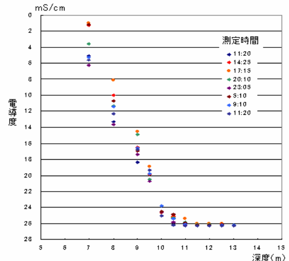
図-8 ボーリング井①の淡水・海水境界の位置と潮位による境界の挙動
