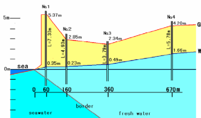
図-6 観測井の水位標高(WL)
