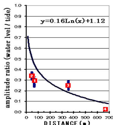
図-7 海洋潮汐影響の距離
