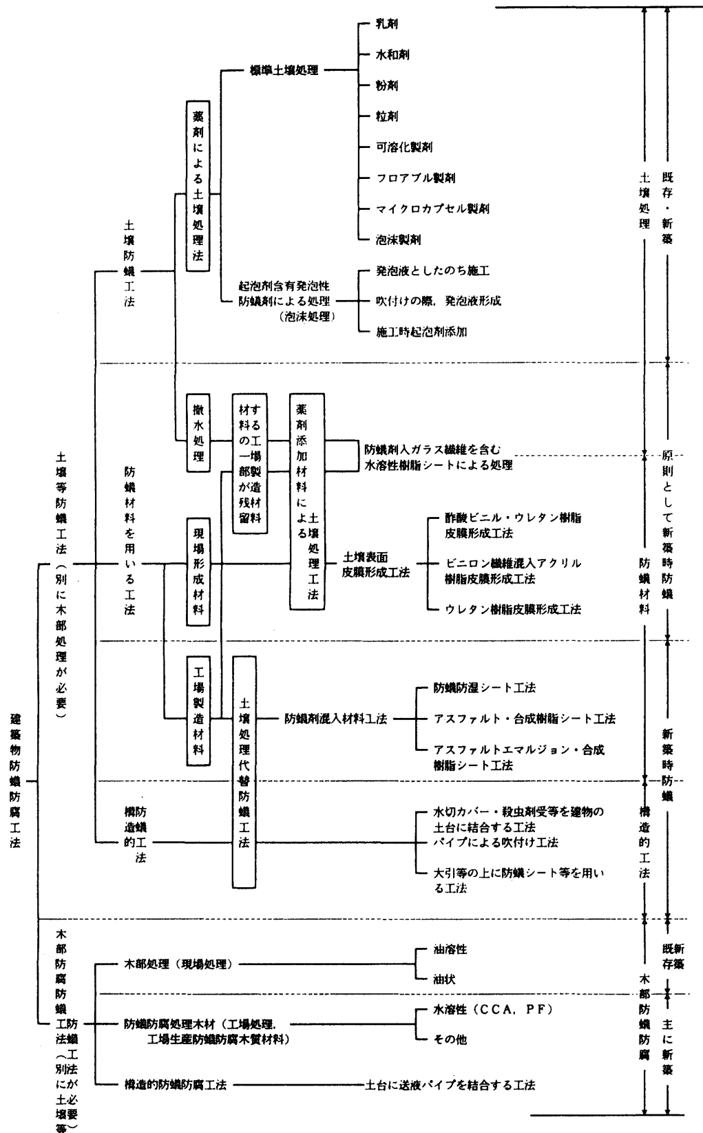
図3 実用化されている建築物防蟻防蝕工法の分類 6)
