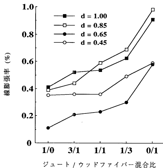
図12 ファイバーの混合比と線膨張率の関係
