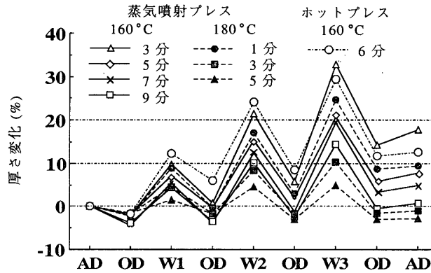
図21 促進劣化処理によるバグスパークルボードの厚さ変化
