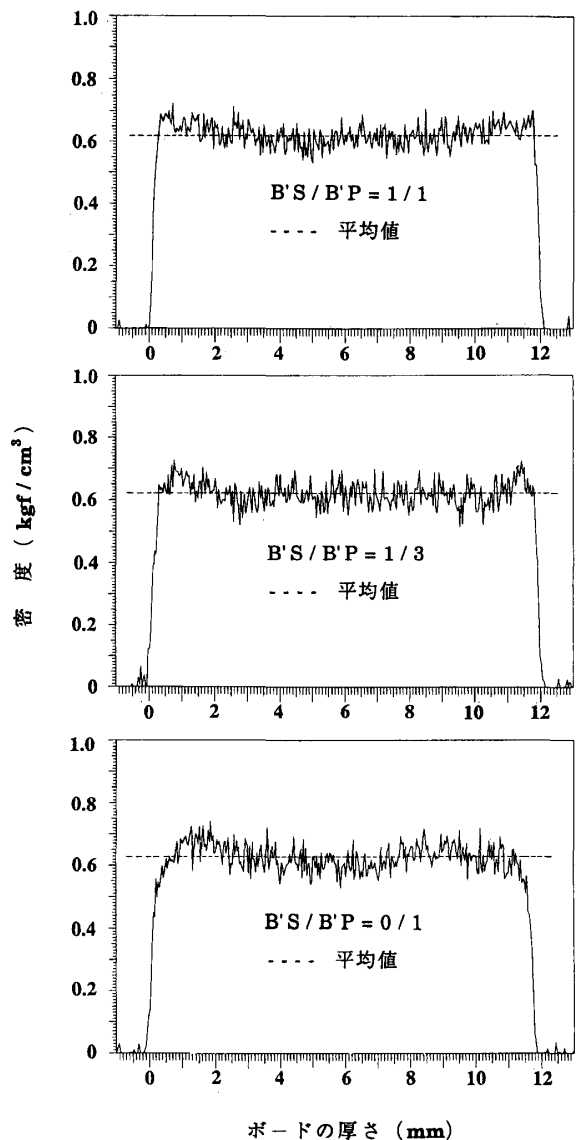
図34 バガス複合ボードの厚さ方向における密度分布 注: B'S: バガスストランド, B'P: バガスパーティクル
