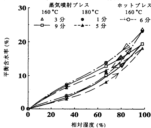
図22 バグスパークルボードの吸湿等温曲線
