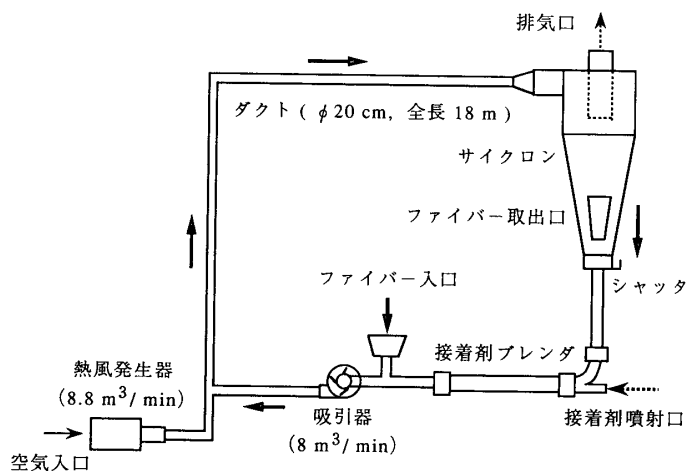
図4 ファイバーの乾燥・接着剤添加の模式図
