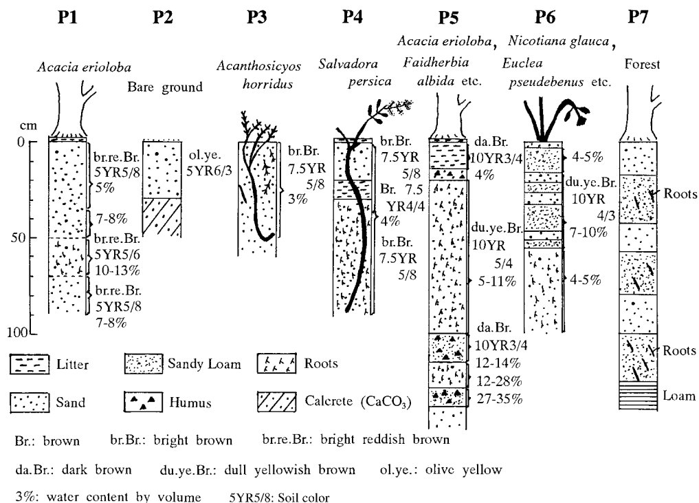
図5 各調査地点 (図4に示した) における土壌断面図
