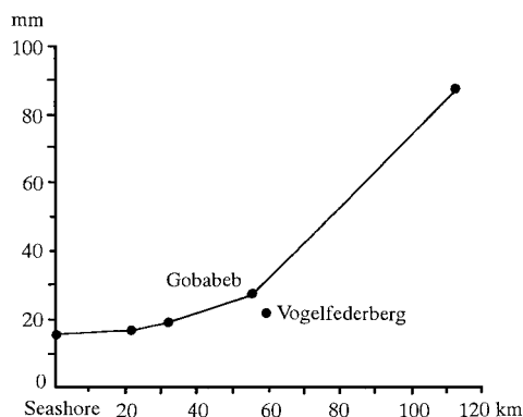
図2 中部ナミビアの海岸からの距離に対する年平均降雨量 [Lancaster et al. 1984]
