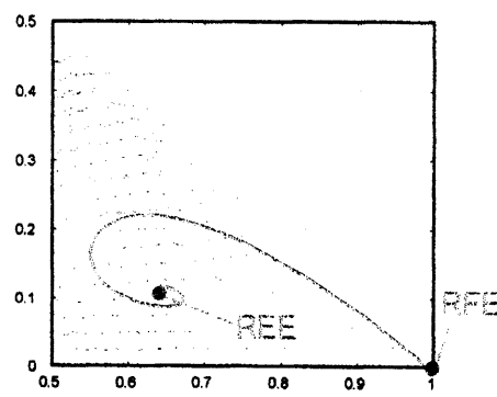
図 2: 方程式系 (3.2) に対するベクトル場と相図. ただし d = 1.2 > \theta のとき.
