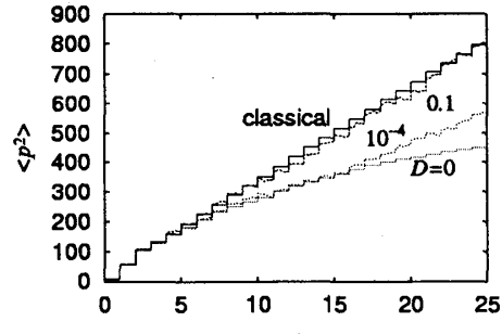
図1 Kicked Rotor での \langle p^2 \rangle 一番上の線が古典力学によるもので一番下が量子力学によるもの。それらの中にある2本は量子+decoherence の場合。上のものが D = 0.1 、下が D = 10^{-4} の結果。
