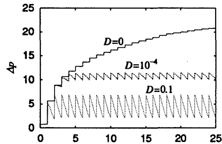
図 2(b) QT の p 方向の幅 \Delta p 一番上の線は D=0 の pure な量子的時間発展の場合。次が D=10^{-4} 、その下が D=0.1 。幅が平衡値に達する時刻は \Delta x の場合とほとんど同じになっている。
