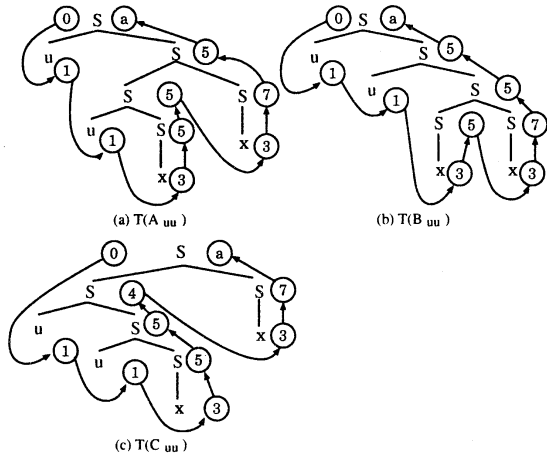
図 1: 入力 uuxx の構文解析木
