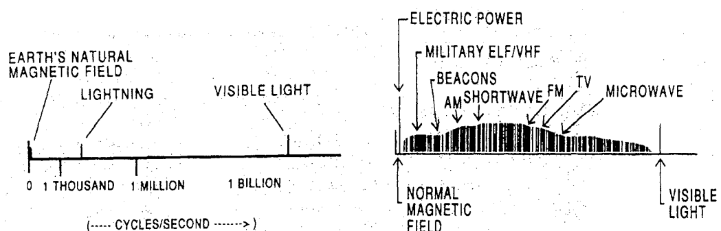
（図 1）自然界の電磁波スペクトル（図 2）人工の電磁波スペクトル （Robert, O. Becker, “Cross Currents”より）
