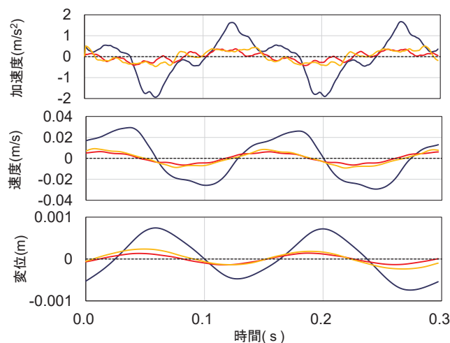
図6 入力加速度3.5 m/s 2 振動数7.0 Hz
