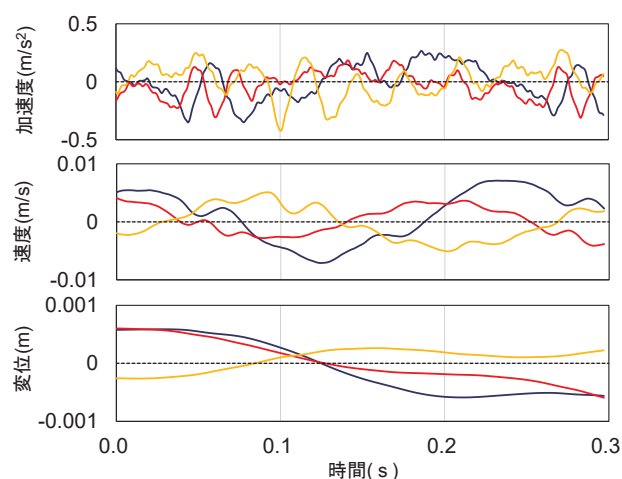
図5 入力加速度2.2 m/s 2 振動数4.5 Hz (青：藁 赤：木 黄：煉瓦 以下同様)
