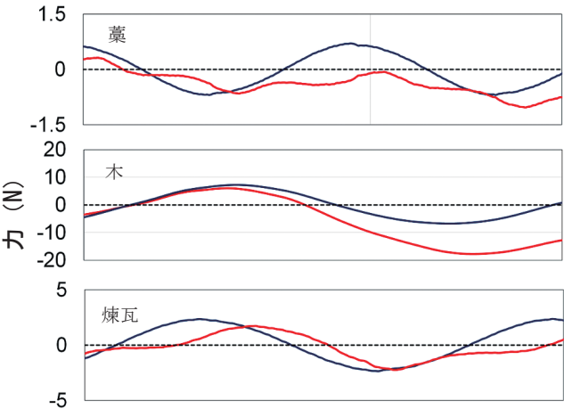
図1 運動方程式における入力と応答の比較 (赤：応答 青：入力)
