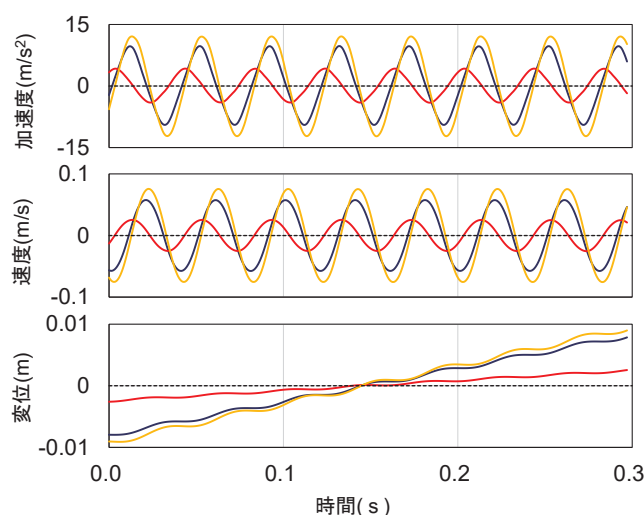
図7 入力加速度3.4 m/s 2 振動数25 Hz
