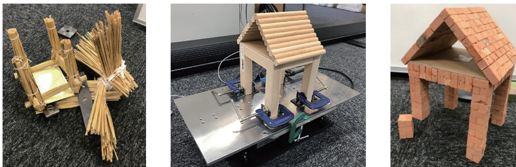
図8 破壊状況（左から藁，木，煉瓦）
