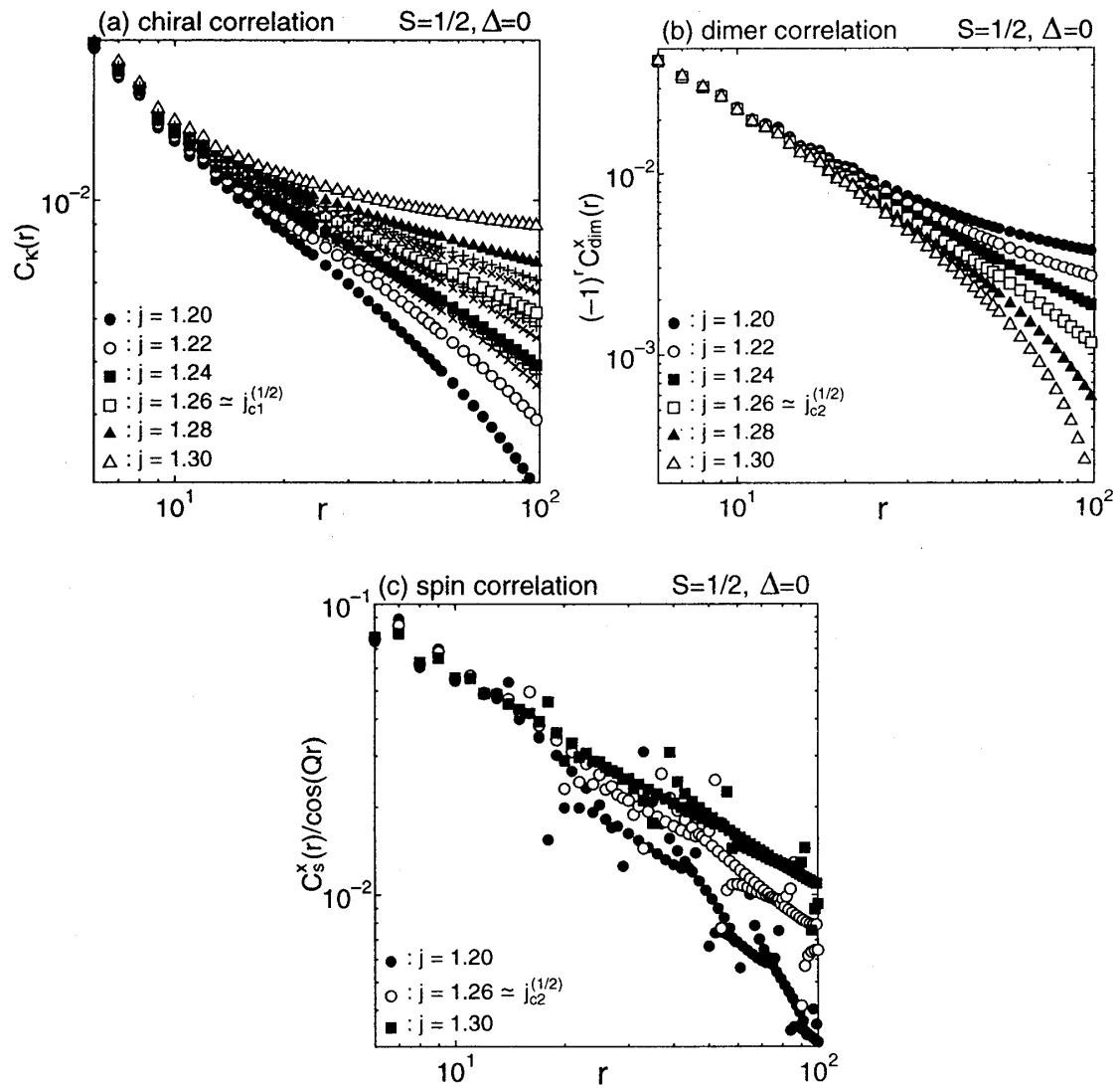
図 1: S = 1/2 XY ( \Delta = 0 ) 模型における相関関数 and various j : (a) カイラル相関関数 C_K(r) ; (b) ダイマー相関関数 (-1)^r C_{\text{dim}}^x(r) ; (c) スピン相関関数 C_s^x(r)/\cos(Qr) .
