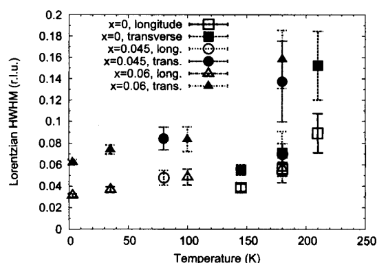
図 1: Q = (1/2 \ 1/2 \ 0)_{tet} , \hbar\omega = 10 meV 周辺での磁気ゆらぎピーク幅の温度依存性。
