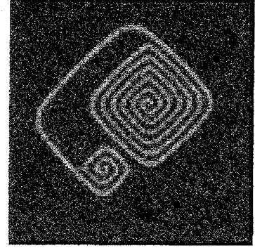
図5 BZ反応モデルCAを時間連続化した微差分方程式の時間発展パターン
