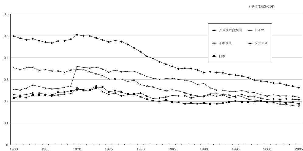
図1 先進国のエネルギー効率、1960-2005年
