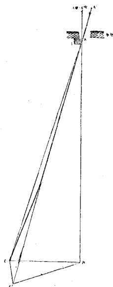
第1圖 隕石落下の經路
