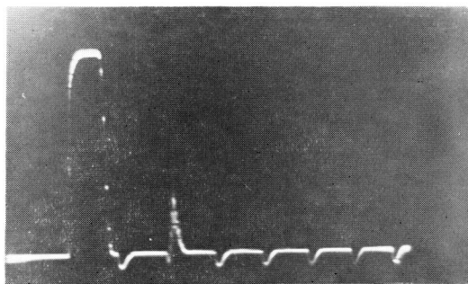
図2-b テストピースのエコーパターン Pulse L. 2.0 T.P. : 送信パルスエコー T. : テストピースのエコー (2cm の距離からのエコー : 卅)
