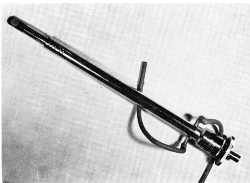
図5 特殊探触子 5 MC 10mmφ (経直腸の水浸法用)
