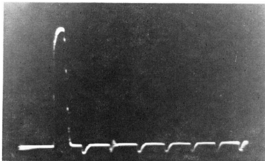
図2-a テストピースのエコーパターン Pulse L. 1.0 T.P. : 送信パルスエコー T. : テストピースのエコー (2cm の感離からのエコー : 卅)
