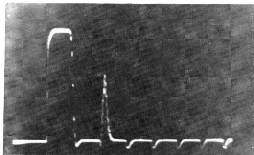
図2-c テストピースのエコーパターン Pulse L. 3.0 T.P. : 送信パルスエコー T. : テストピースのエコー (2cm の距離からのエコー : 卅)
