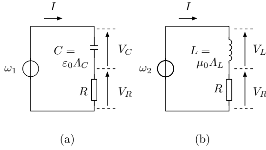
図 1: コンデンサとコイルのリアクタンス測定により \varepsilon_0 , \mu_0 を定め, 光速 c_0 を求める.
