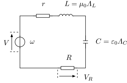
図 2: LC 共振回路による c_0 の測定。
