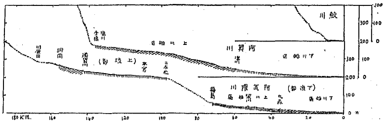
第一圖 河川の縦断面と通航區
