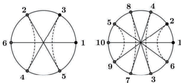
図 1: 素数 7 の絵 (左) と, 素数 11 の絵 (右)
