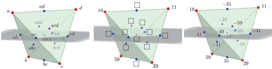
図 6: (\mathbb{Z}/120\mathbb{Z})^\times の立体射影, その計算パズルと, 計算パズルの解
