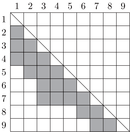
図 1 h = (4, 5, 7, 7, 7, 8, 9, 9, 9) のときの絵
