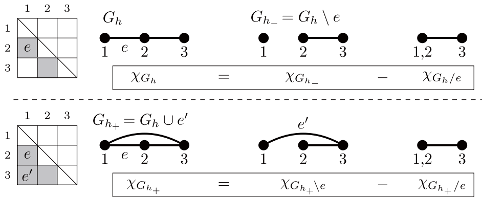
図 2 2つの deletion-contraction
