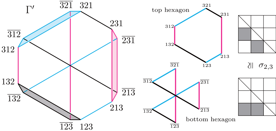
図 4 GKM 的なデータ \Gamma' の絵
