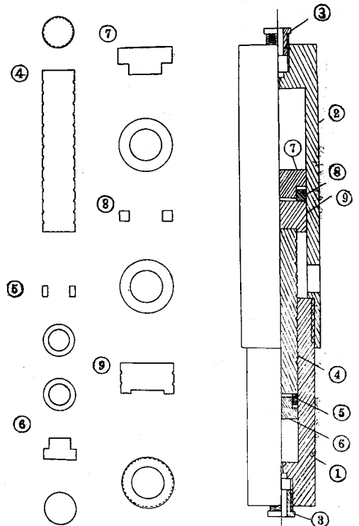
高圧用ピストン設計図
