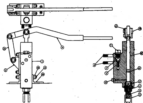
吸上ポンプ設計図
