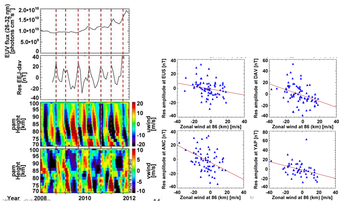
図 3.5.6 (左)SOHO 衛星で観測された太陽極端紫外線(26-32 nm)フラックス、赤道域磁場 (DAV) における Res-EEJ 振幅変動とインドネシアのパンプクに設置された MF レーダーから見積もられた東西・南北風速変動。(右)赤道域における 4 つの観測点(EUS、DAV、ANC、YAP) で観測された Res-EEJ 振幅とインドネシアのパンプク上空の高度 86km における東西風速との相関関係。
