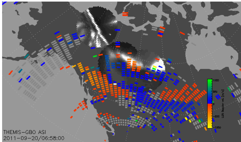
図 3.3.3 2011 年 9 月 20 日に電離層レーダー（SuperDARN レーダー）と全天イメージャで取得された電離圏プラズマ速度とオーロラ画像の重ね描きの例。このように、UDAS では、地図上に多種多様な 2 次元データを描画することを目指している。
