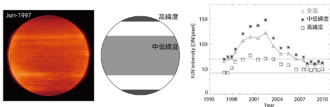
図 3.5.2 (左)1997 年 6 月の 1 カ月平均画像(SOHO/EIT 304A による)。(中)高緯度領域(緯度 60 度以上)と中低緯度(緯度 0 度以上 30 度未満)の模式図。(右)高緯度領域(□)、中低緯度領域(*)、太陽全面(△)での極端紫外線強度の長期変動。2008 年ごろでは、高緯度域の強度が 1997 年ごろに比べて明るい一方で、中低緯度域や全面では暗くなっている。
