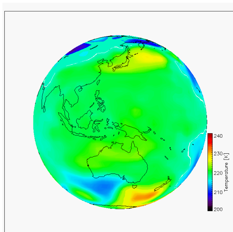
図 3.3.4 九州大学の気象大循環モデルによって計算された 2009 年 1 月 1 日 200hPa 高度における大気の温度分布。UDAS により作成。
