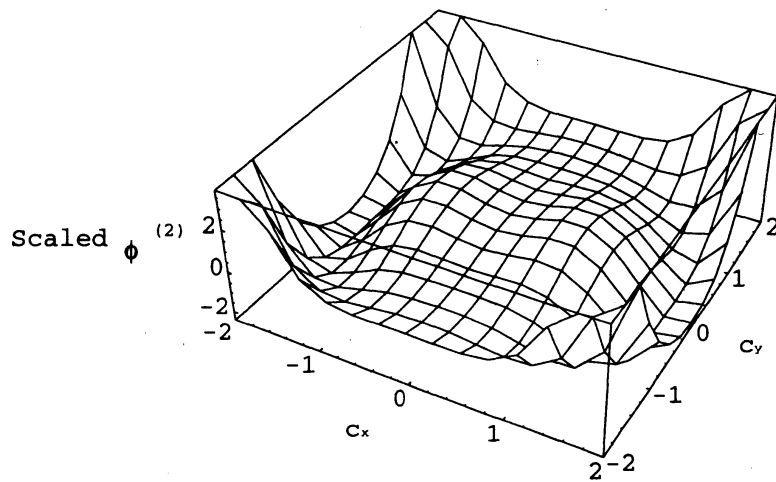
図 2: Sonine 7 次近似の剛体球分子の非線形摂動解 \phi^{(2)}(c) 。無次元量 mJ_x^2/n^2\kappa^3T^3 でスケールされている。 c_z = 0 とおいた。
