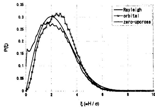
図 15: E(k) \propto k^{-4} スペクトルを有する波形の波高分布 (個々波分割はゼロアップクロス法およびオービタル法)
