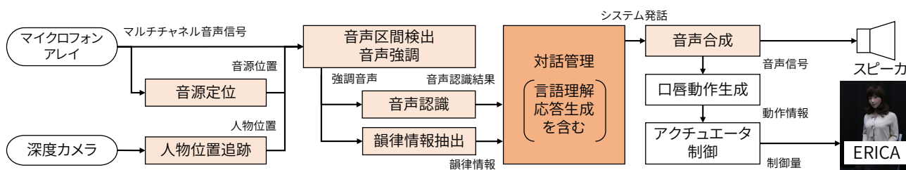
図2 アンドロイド ERICA の音声対話システムの構成 (傾聴対話システムは「対話管理」の内部に相当する)
