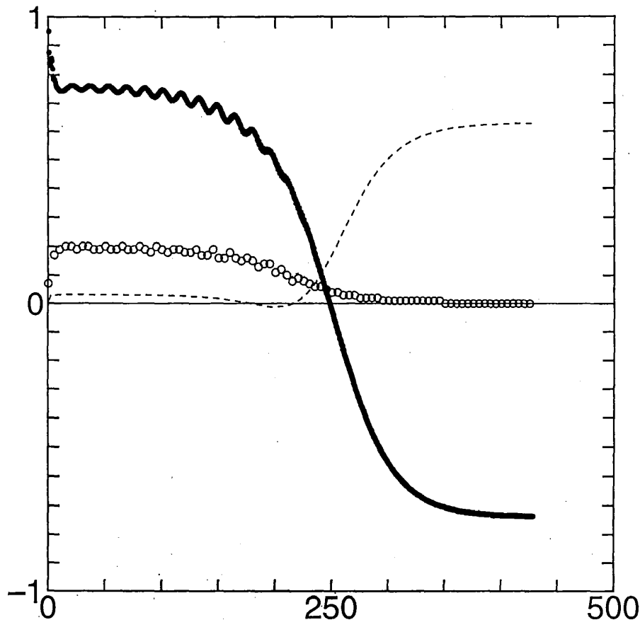
図2 J = 1.0 , \Gamma = 0.2 , H = 1.0 , a \neq 0.0 における磁化とボーズ粒子数の時間変化。破線はエネルギーの時間変化。
