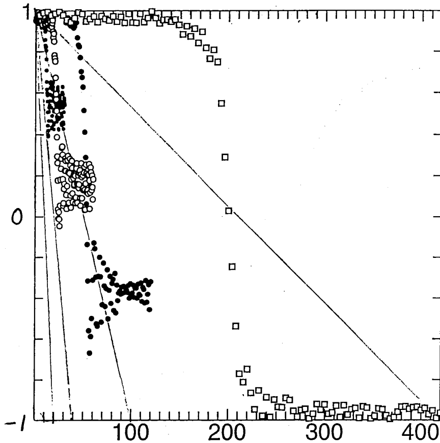
図1 J = 1.0 , \Gamma = 0.5 , H = 1.0 , a = 0.0 , N = 2 における磁場の変化速度化と磁化の時間変化。実線は H(t) を表し、 \bullet , \circ , \bullet , \square はそれぞれの H(t) での磁化変化。
