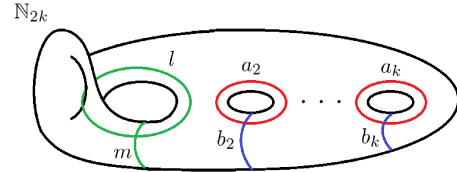
図 7: N_{2k} の基本群 \pi_1(N_{2k}) の生成元
