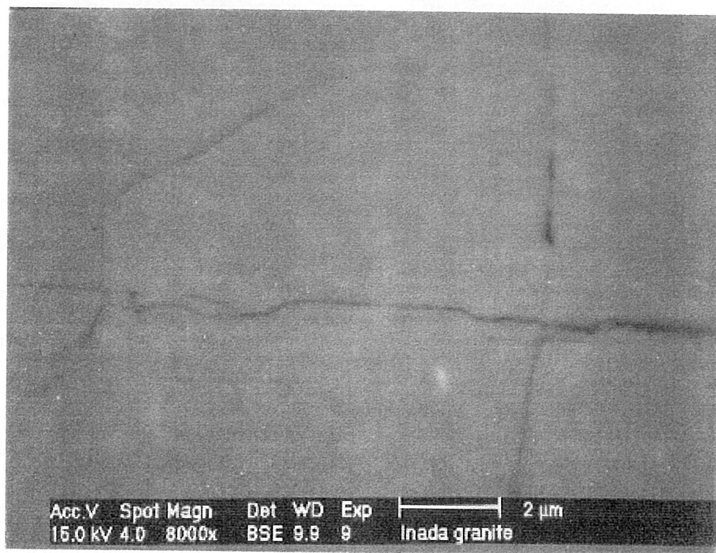
Fig. 2-7 SEM images of Inada granite
