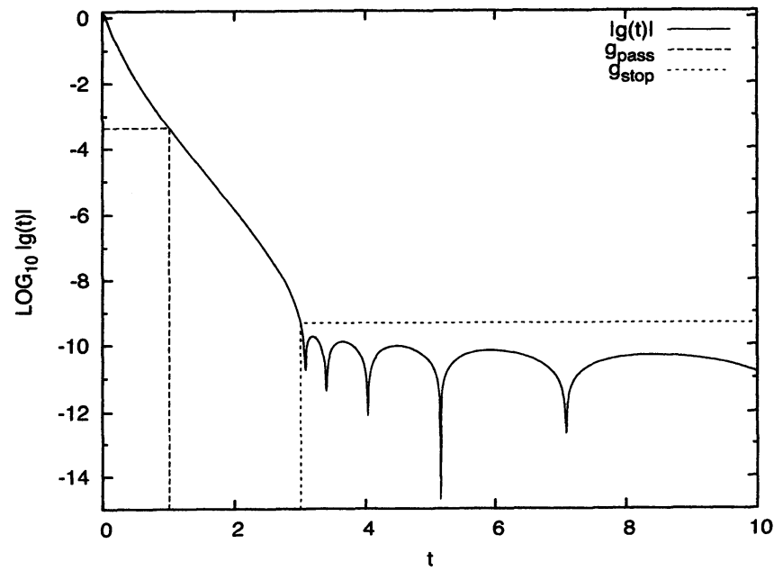
図 4: フィルタ (その 2) の伝達関数 |g(t)| (対数値) ( n = 16 , \mu = 3 , g_{\text{pass}} = 4.2\text{E-}4 , g_{\text{stop}} = 4.7\text{E-}10 )
