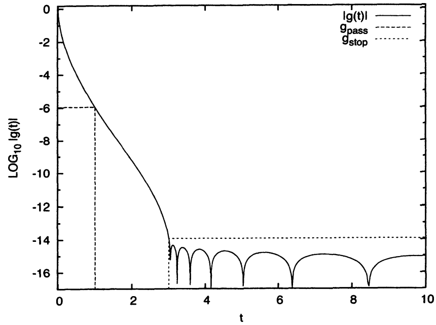
図 3: フィルタ (その 1) の伝達関数 |g(t)| (対数値) ( n = 16 , \mu = 3 , g_{\text{pass}} = 1.07\text{E-}6 , g_{\text{stop}} = 1.16\text{E-}14 )
