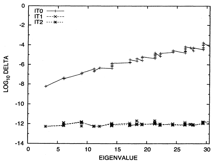
図 6: 例題 1 : 近似対の残差のノルム \Delta (区間 [0, 30] , m=300 )
