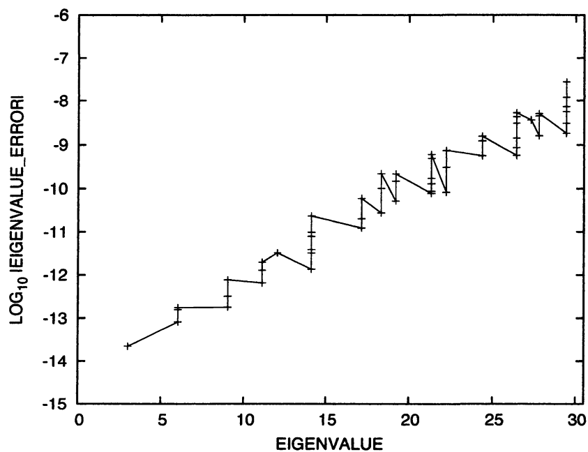
図 10: 例題 2 : 近似固有値の真値からの誤差の分布 ( m=300 , 閾値 2.12\text{E-}4 )
