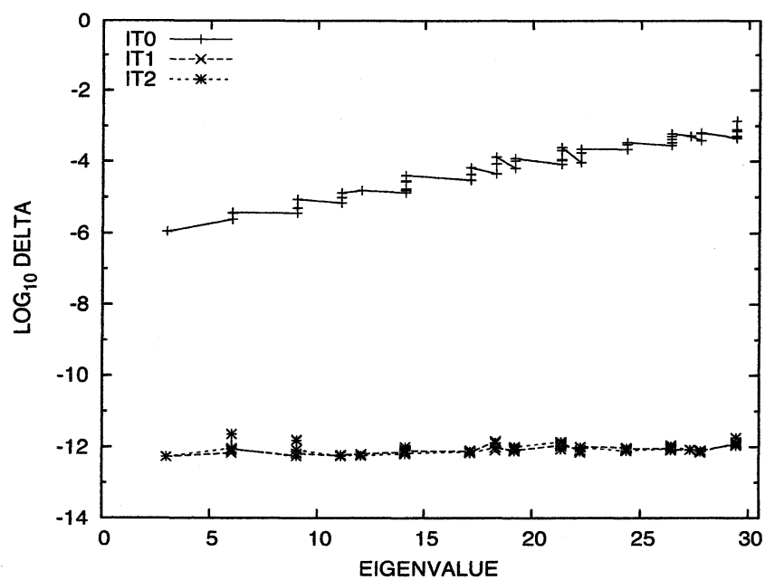
図 9: 例題 2 : 近似対の残差のノルム \Delta (区間 [0, 30] , m=300 )
