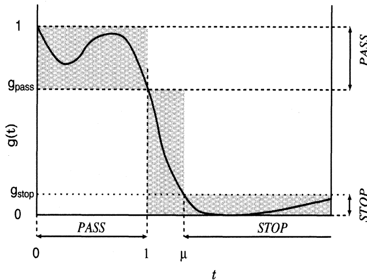
図 2: フィルタの伝達関数 g(t) の概形図（下端付近の固有値に対する）
