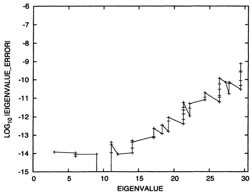
図 7: 例題 1: 近似固有値の真値からの誤差の分布 ( m=300 , 閾値 5.33\text{E-}7 )
