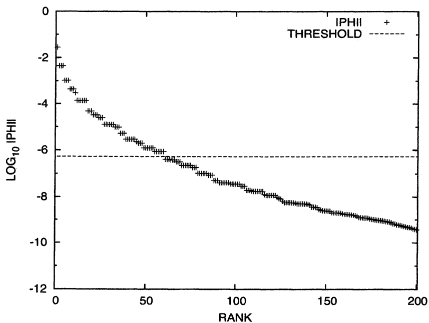
図 5: 例題 1 : |\phi| の値の分布 ( m=300 , 閾値 5.33\text{E-}7 )
