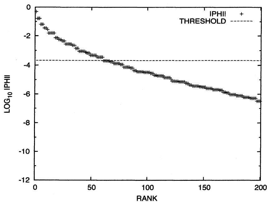
図 8: 例題 2 : |\phi| の値の分布 ( m=300 , 閾値 2.12E-4 )
