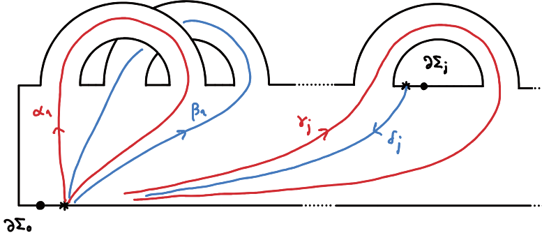
図 1: 基本亜群 \mathcal{G} の自由生成系 \mathcal{C} .
