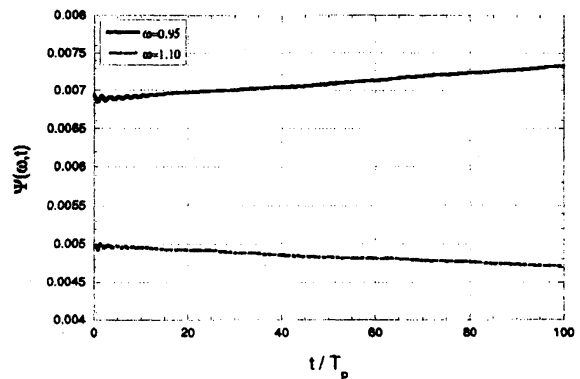
図 4: \omega = 0.95 と 1.10 における \Psi(\omega) の時間変化の一例 (JONSWAP, \cos^2 \theta , E = 0.003 )
