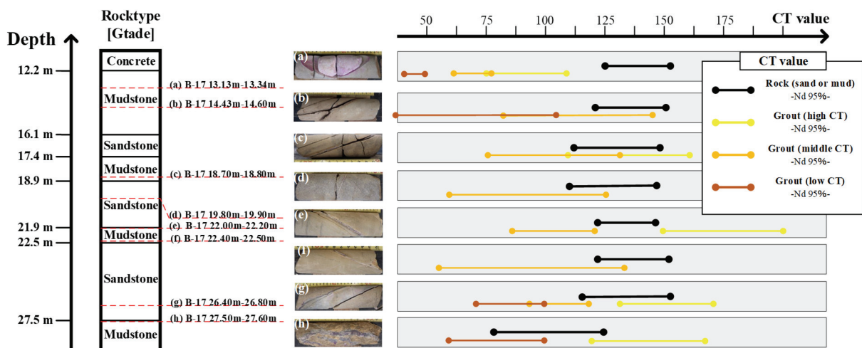
図-10 \mu X線CT撮影地点でのCT値の分布
