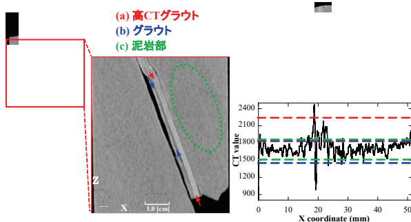
(b) 18.70 m 地点 (18.70~18.80 m)
