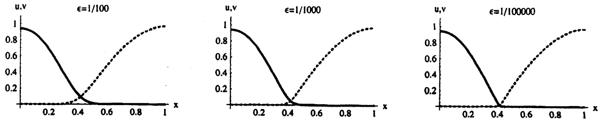
図 1: \varepsilon による (3.1) の解の形状の変化. f(u) = u(1-u) , g(v) = v(1-v) , d_1 = 0.1 , d_2 = 0.1 のときの u, v を実線 (青), 破線 (赤) で描いている.
